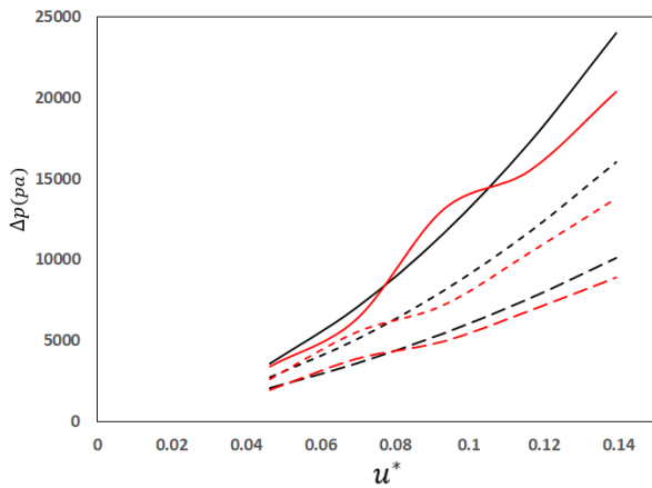
(a) Da = 10^{-6}
